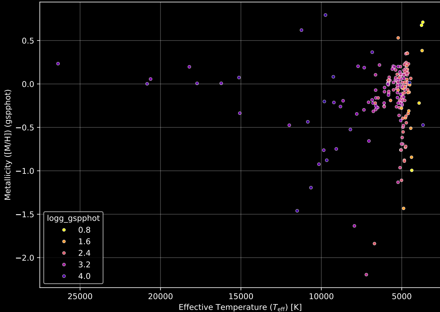
APOGEE DR17 Field: [101+04] Stellar Population Parameters (n= 194)
